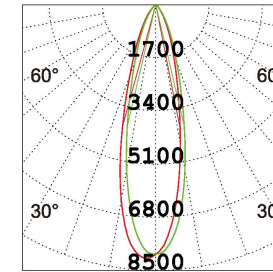
3×10W 3000K 24 °
