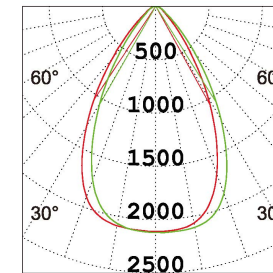
3×10W 3000K 60 °
