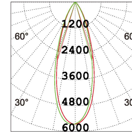
3×10W 3000K 36 °
