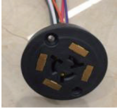
7pin NEMA
