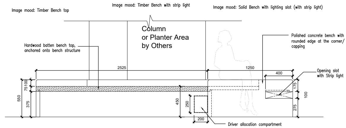
ELEVATION B
