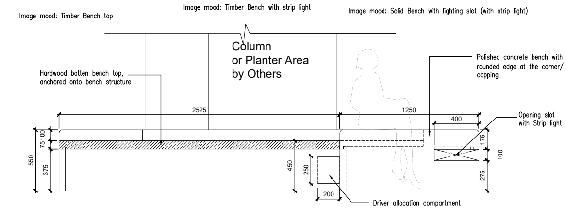
ELEVATION B
